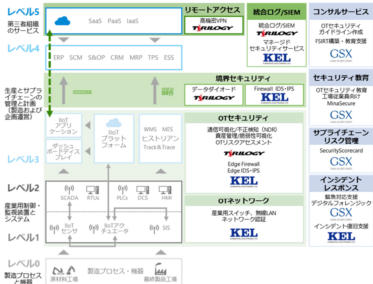
Purdueモデル
